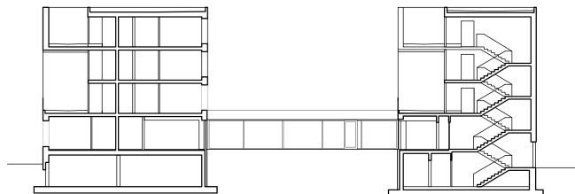
Querschnitt 1. Bauabschnitt
