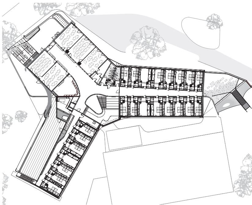
Grundriss Obergeschoss
