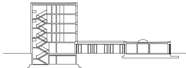
Längsschnitt 2. Bauabschnitt
