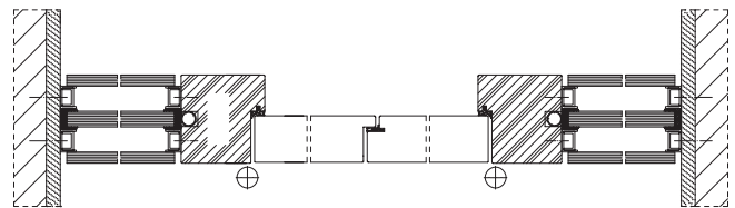
Horizontalschnitt
