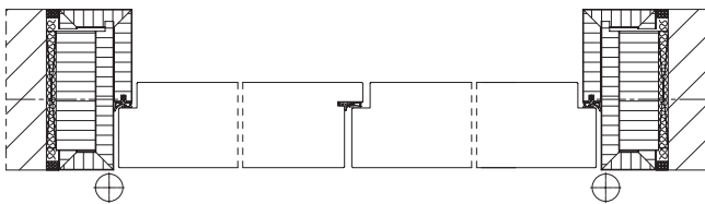
Horizontalschnitt
