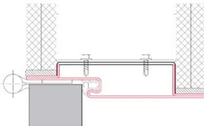
Zargenschnitt (2)
