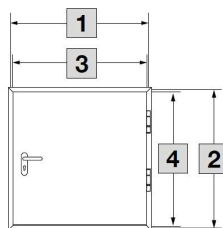
Klappe 2-seitig gefälzt
