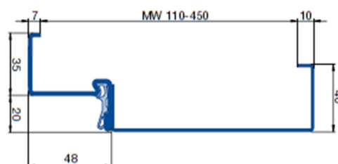
Eckzarge mit Ergänzungszarge
