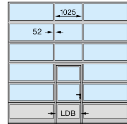
ALR F42, ALR F42 Thermo, ALR 67 Thermo Schlüpftüranordnung Mitte
