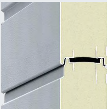
Thermisch getrennte Lamellen beim SPU 67 Thermo
