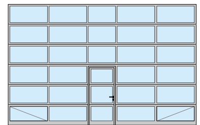
ALR F42, ALR F42 Thermo, ALR 67 Thermo Schlüpftüranordnung Mitte Vollverglasung
