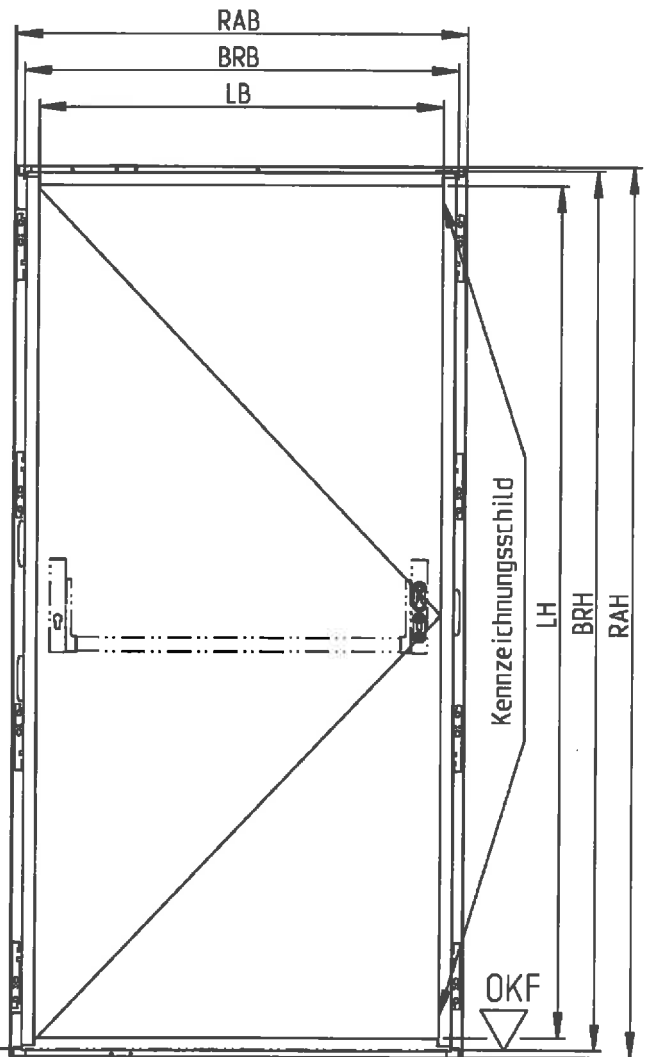
Ansicht Schließseite
