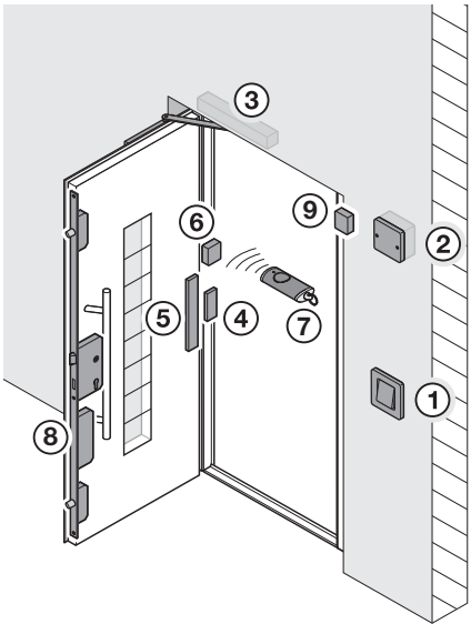
S5 Ecturn Smart (KÜ)
