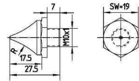
Sicherungsbolzen wahlweise
