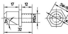
Sicherungsbolzen wahlweise
