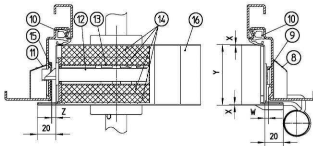
Horizontalschnitt Dünnfalztür
