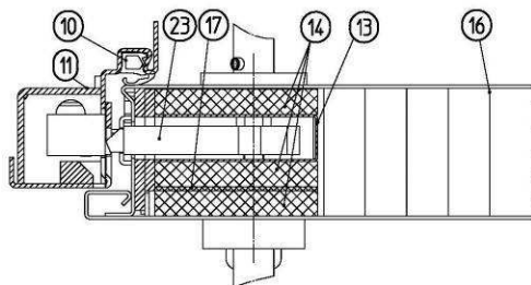
Horizontalschnitt Dickfalztür
