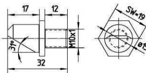
Sicherungsbolzen wahlweise
