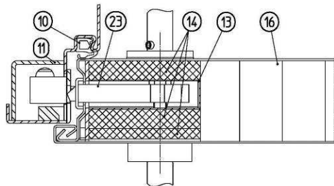
Horizontalschnitt Dickfalztür
