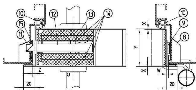
Horizontalschnitt Dünnfalztür
