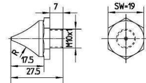
Sicherungsbolzen wahlweise
