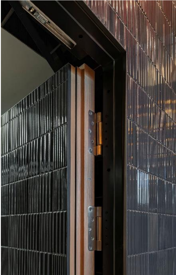
Bild 4: Robuste und formstabile Stahlzargen zeichnen sich durch exakte Profilgeometrie und hohe Formstabilität aus.
